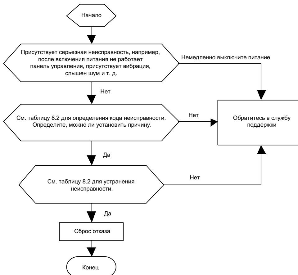
Рисунок 10.2. Блок-схема диагностики неисправностей
