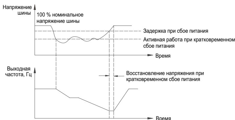
Рисунок 8.12.1. Схема безостановочной работы при кратковременном сбое питания
