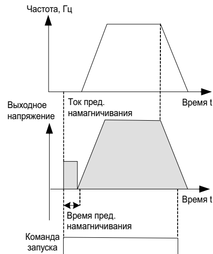
Рисунок 8.3.2. Временная диаграмма для режима предварительного намагничивания с последующим пуском
