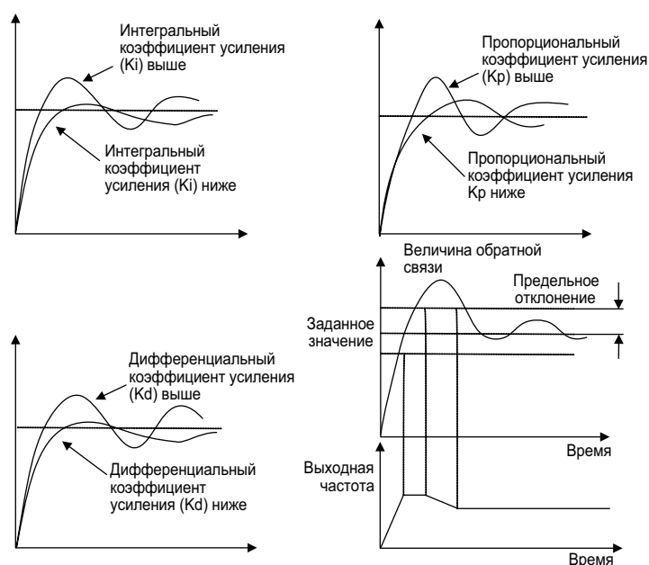
Рисунок 8.2.8. Влияние параметров ПИД-регулятора
