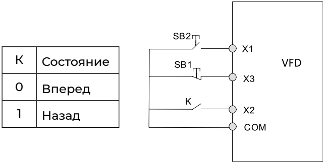
Рисунок 8.1.4. Режим трехпроводного управления 2
