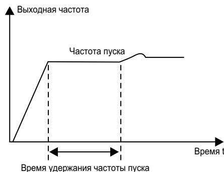
Рисунок 8.3.1. Временная диаграмма для режима пуска с заданной частотой пуска
