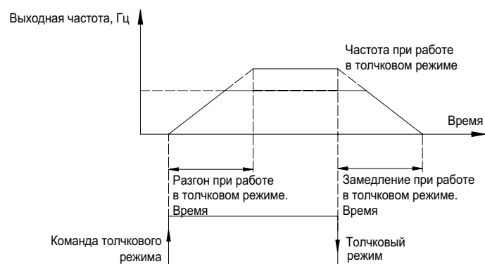
Рисунок 8.13.1. Принципиальная схема работы в толчковом режиме
