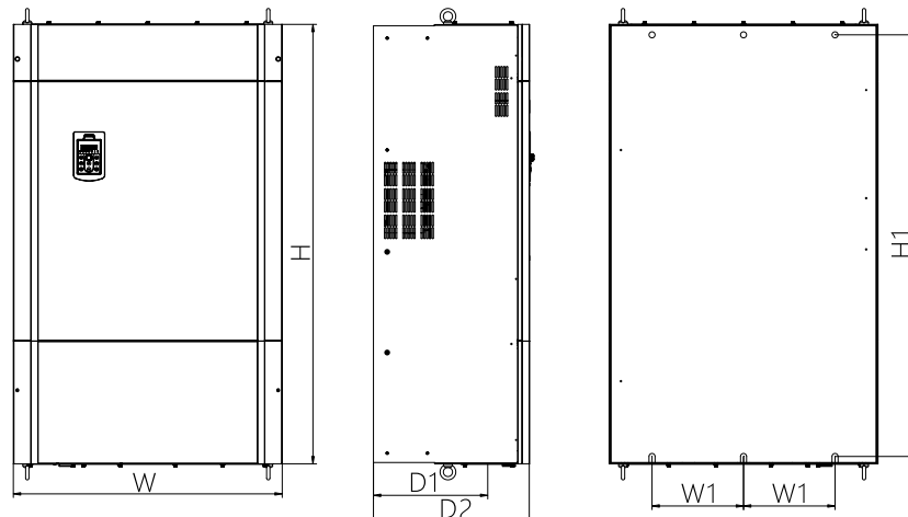
Рисунок 5.5. Внешний вид и габаритные размеры NVF2G-S-315/TS4–NVF2G-S-400/TS4
