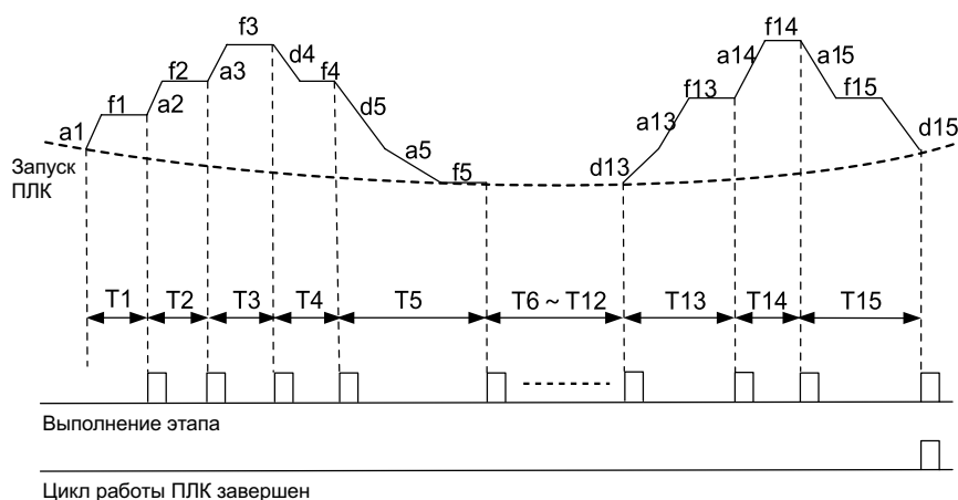
Рисунок 8.2.3. Принципиальная схема использования простого ПЛК в качестве источника основной частоты
