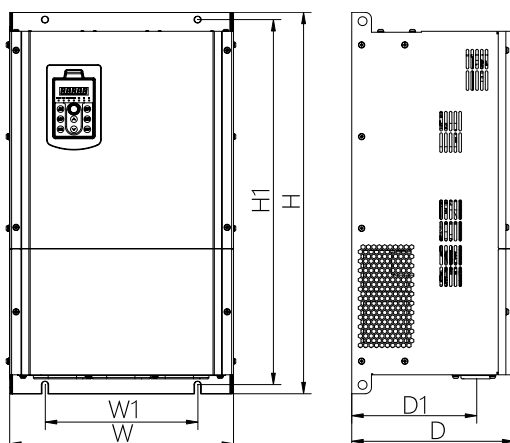
Рисунок 5.3. Внешний вид и габаритные размеры NVF2G-S-30/PS4–NVF2G-S-75/PS4
