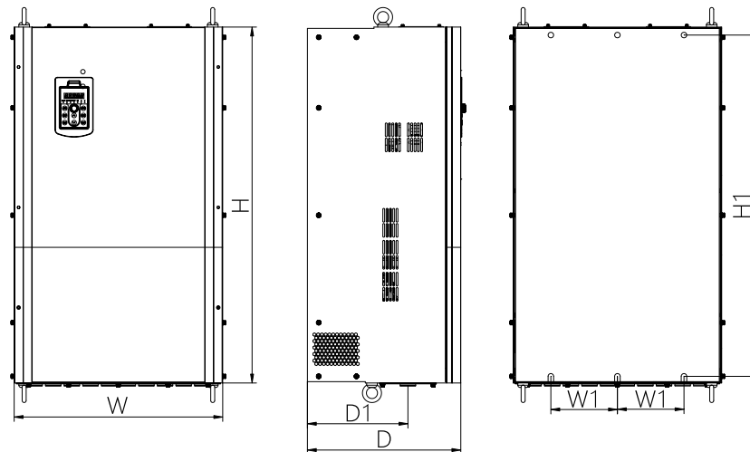
Рисунок 5.4. Внешний вид и габаритные размеры NVF2G-S-75/TS4–NVF2G-S-315/PS4
