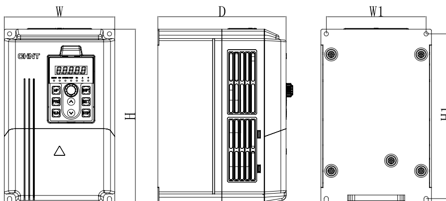
Рисунок 5.1. Внешний вид и габаритные размеры NVF2G-S-1.5/PS4–NVF2G-S-11/PS4
