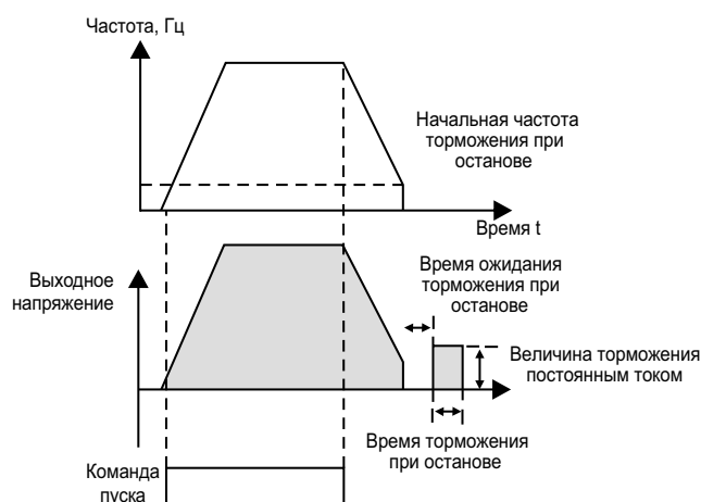
Рисунок 8.3.6. Временная диаграмма для режима останова с заданным временем торможения в комбинации с торможением постоянным током
