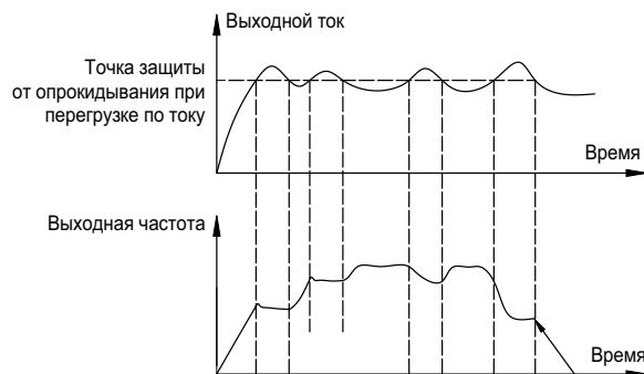
Рисунок 8.7.1. Принципиальная схема работы функции защиты от опрокидывания при перегрузке по току
