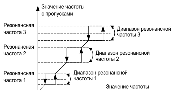
Рисунок 8.14.1. Схема резонансного пропуска частот
