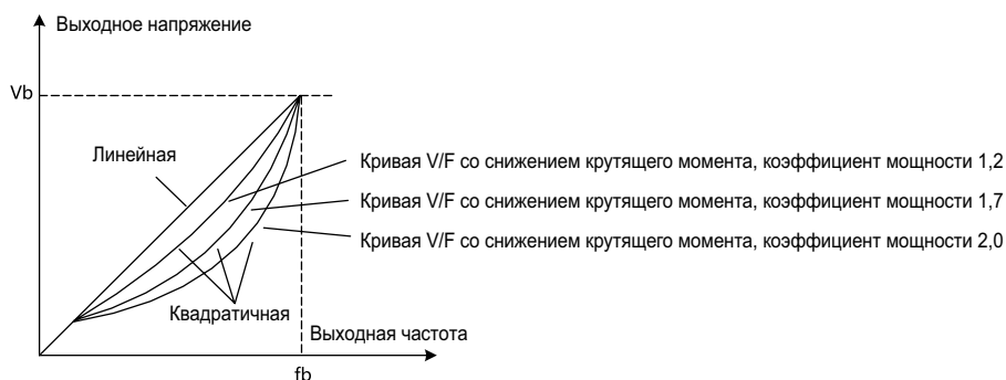
Рисунок 8.5.3. Кривая V/F со снижением крутящего момента
