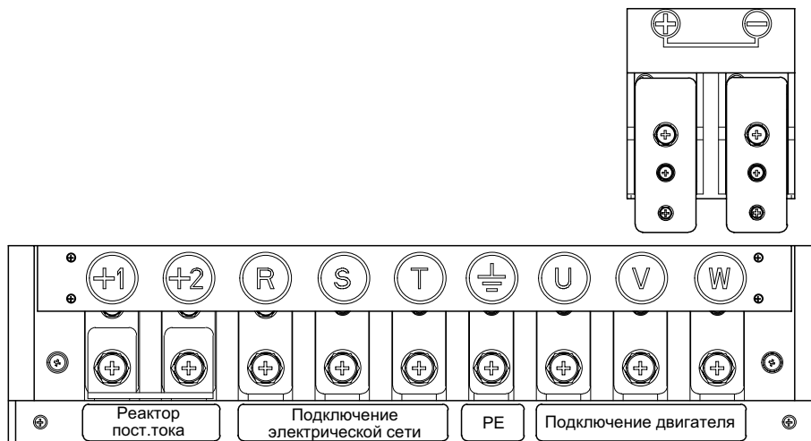
Рисунок 4.10. Силовые клеммы NVF2G-S-160/TS4-315/PS4
