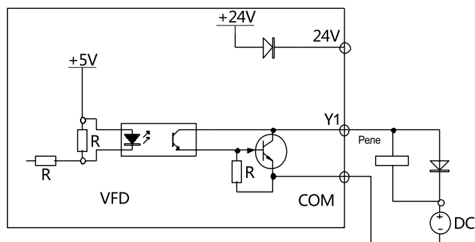
Рисунок 4.18. Схема подключения клеммы многофункционального выхода, режим 2
