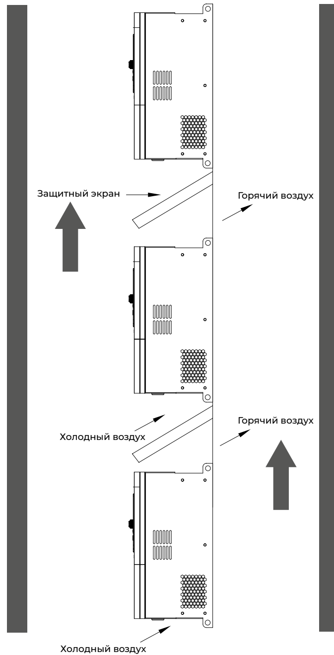
Рисунок 2.2. Вертикальная установка нескольких преобразователей частоты
