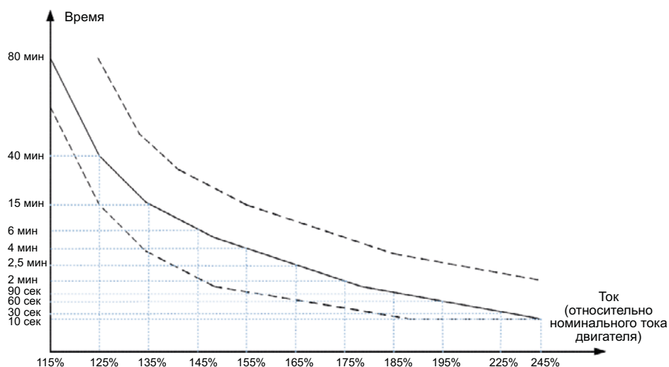
Рисунок 8.9.1. Графики обратной зависимости функции защиты двигателя от перегрузки от времени
