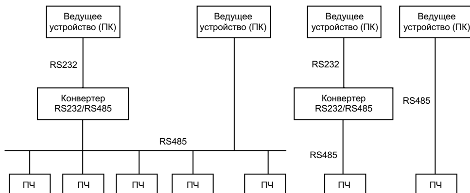
Рисунок 9.1.1. Принципиальная схема сетевого подключения преобразователя частоты
