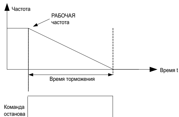
Рисунок 8.3.4. Временная диаграмма для режима останова с заданным временем торможения
