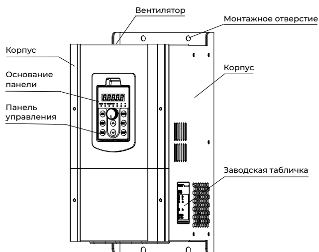
Рисунок 4.2. Внешние компоненты NVF2G-S-11/TS4-NVF2G-S-30/PS4
