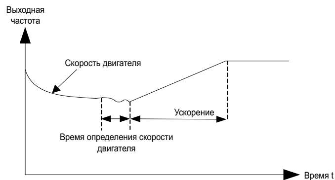
Рисунок 8.3.3. Временная диаграмма для режима повторного запуска после отслеживания скорости
