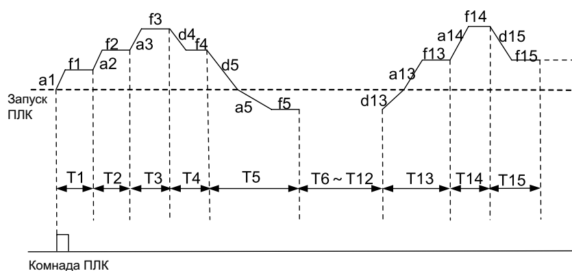
Рисунок 8.2.5. Сохранение конечного значения после одного цикла при использовании простого ПЛК
