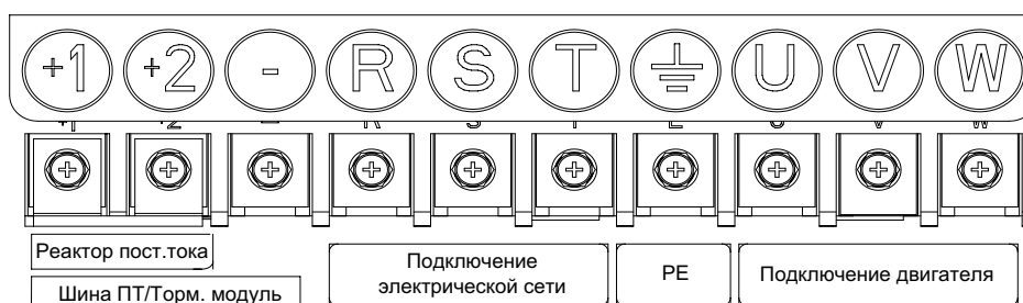
Рисунок 4.9. Силовые клеммы NVF2G-S-110/TS4-160/PS4
