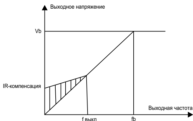
Рисунок 8.5.1. Линейная кривая V/F
