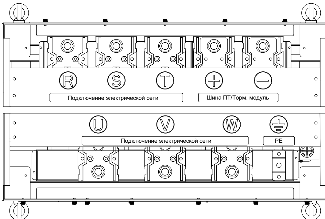
Рисунок 4.11. Силовые клеммы NVF2G-S-315/TS4-400/TS4
