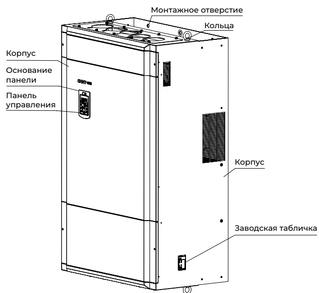
Рисунок 4.5. Внешние компоненты NVF2G-S-315/TS4–NVF2G-S-400/TS4
