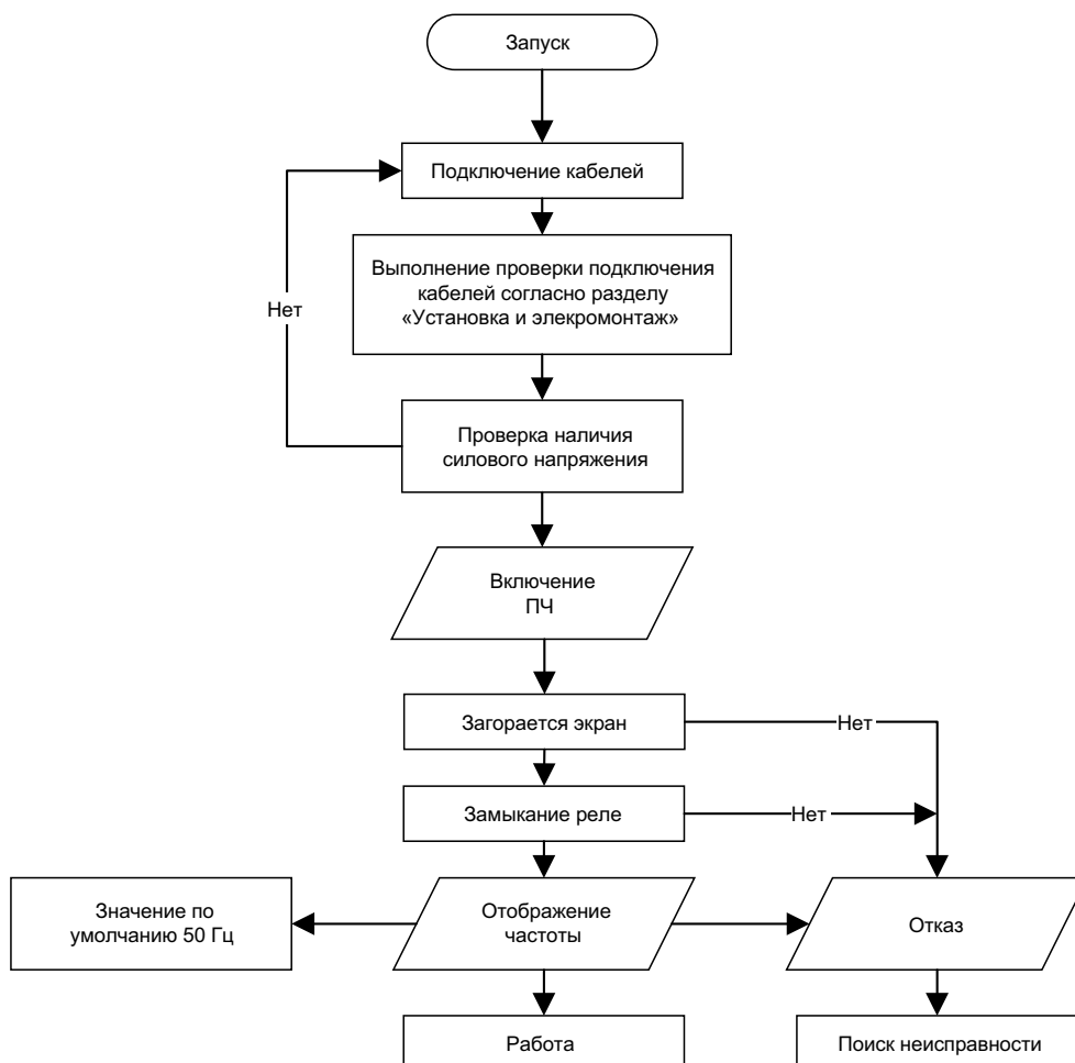
Рисунок 6.1. Последовательность включения питания преобразователя частоты
