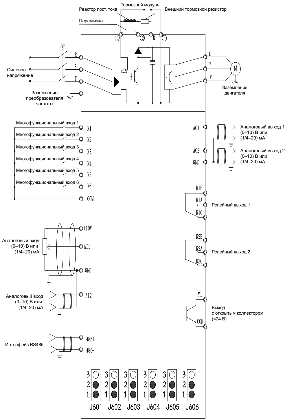
Рисунок 4.12 Схема подключения NVF2G-S-1.5/PS4-NVF2G-S-400/TS4
