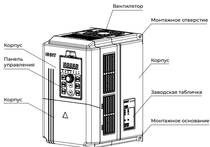
Рисунок 4.1. Внешние компоненты NVF2G-S-1.5/PS4-NVF2G-S-11/PS4
