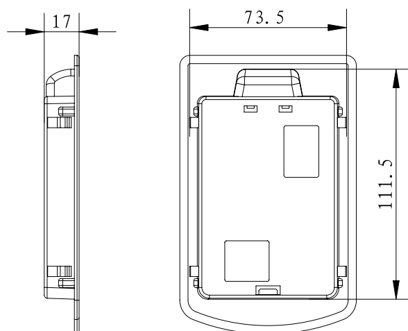
Рисунок 5.7. Монтажное основание панели управления
