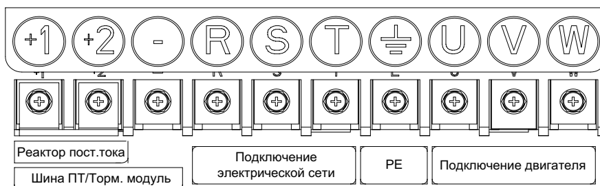
Рисунок 4.8. Силовые клеммы NVF2G-S-45/TS4-110/PS4
