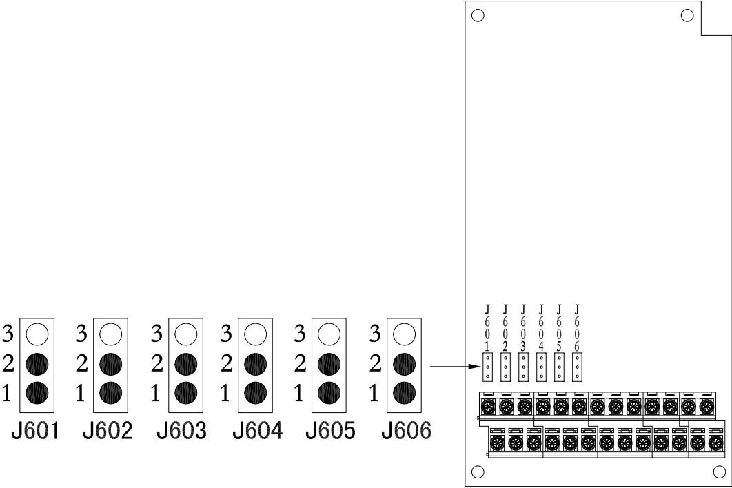
Рисунок 4.13. Положение перемычек
