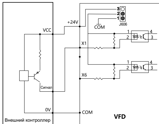
Рисунок 4.15. Схема подключения для логики PNP
