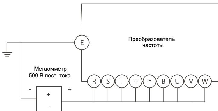
Рисунок 10.1. Измерение сопротивления изоляции силовой цепи
