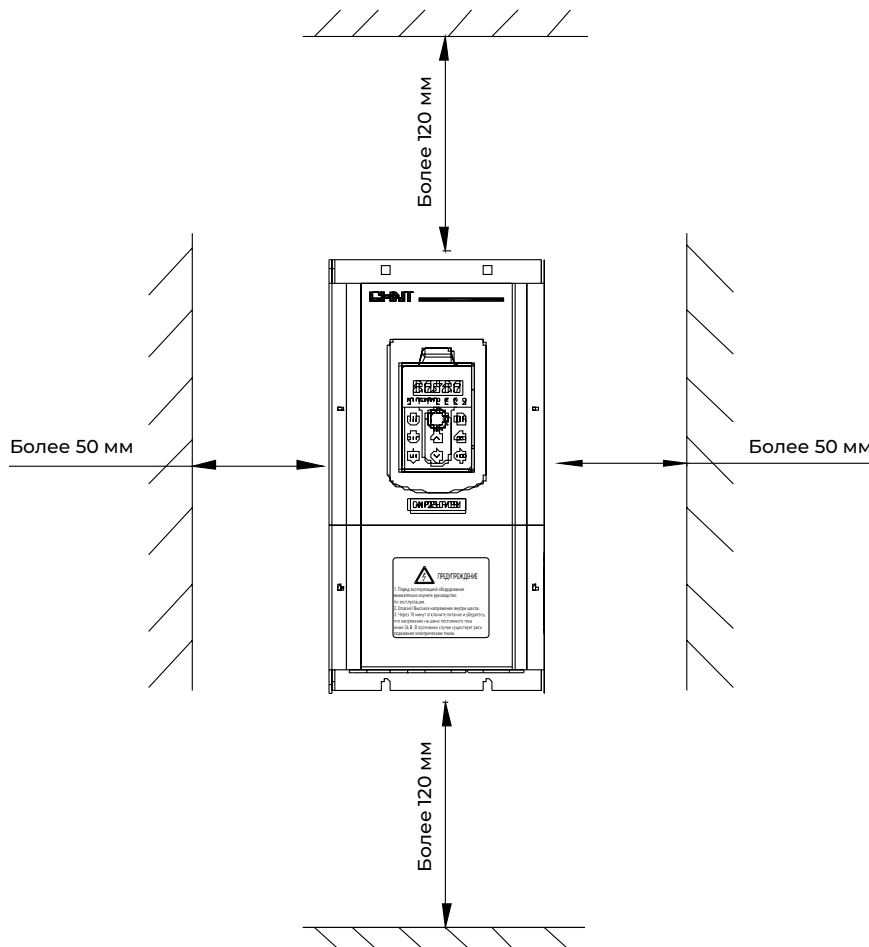
Рисунок 2.1. Схема установки преобразователя частоты
