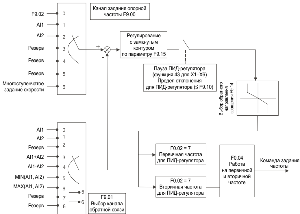
Рисунок 8.2.7. Принципиальная схема использования ПИД-регулятора в качестве источника основной частоты
