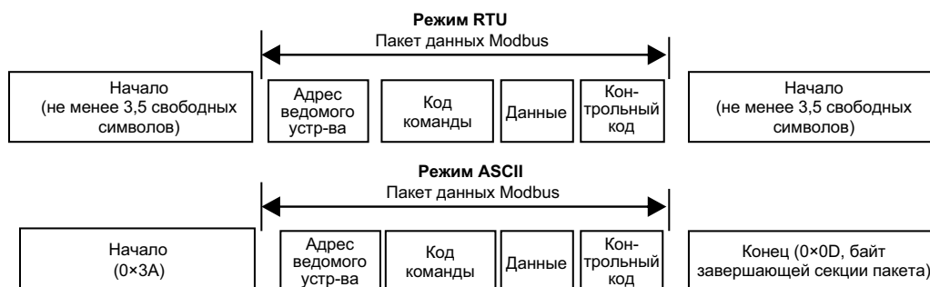
Рисунок 9.4.1. Формат протокола Modbus
