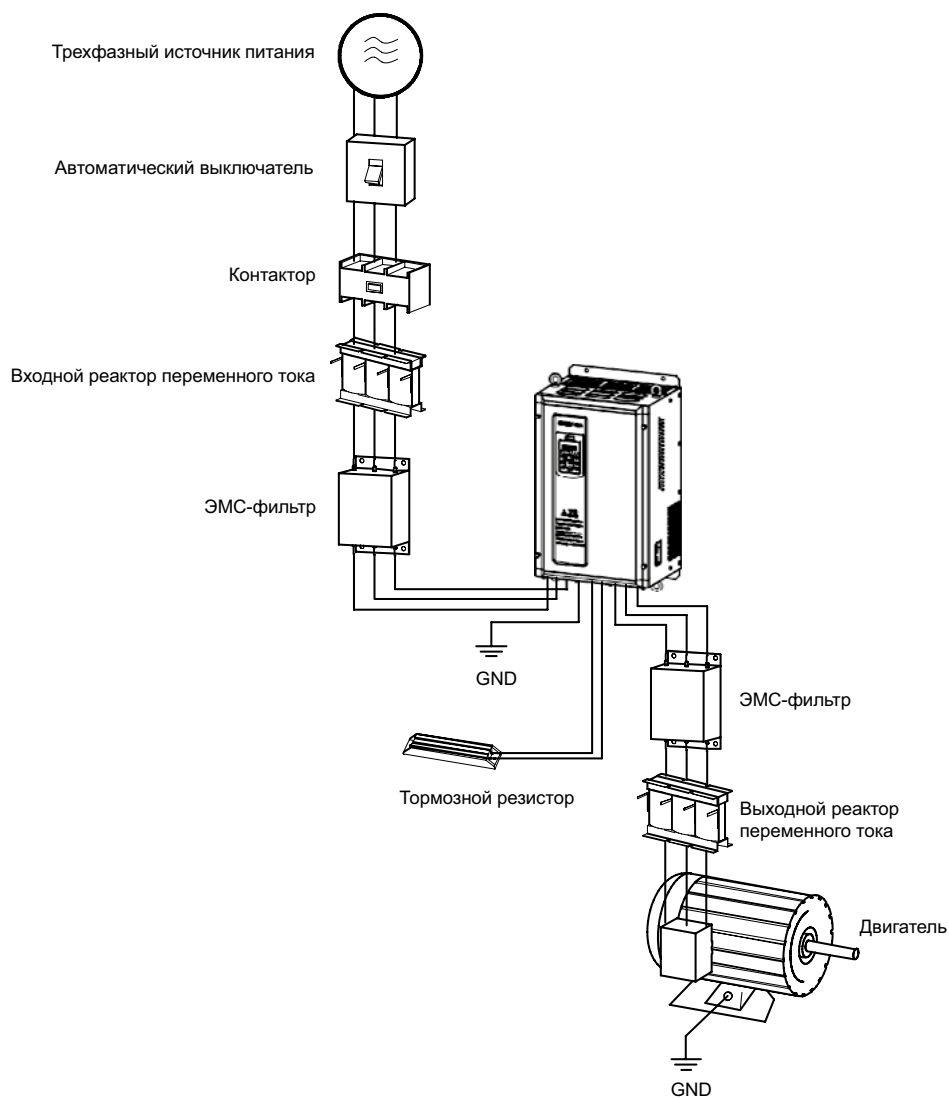
Рисунок А.1. Схема подключения изделия и периферийных устройств
