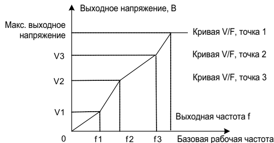
Рисунок 8.5.2. Многоточечная кривая V/F
