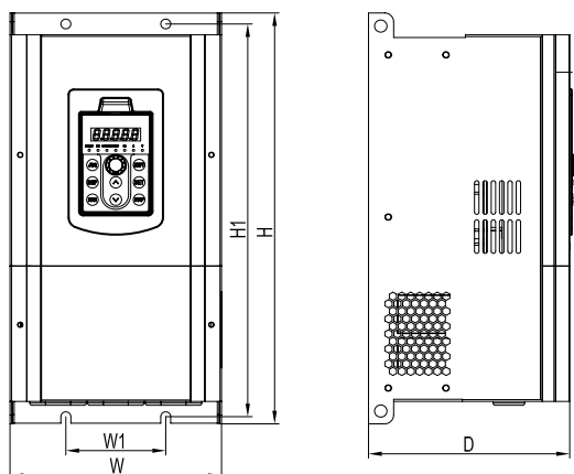
Рисунок 5.2. Внешний вид и габаритные размеры NVF2G-S-11/TS4–NVF2G-S-30/PS4
