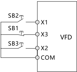
Рисунок 8.1.3. Режим трехпроводного управления 1
