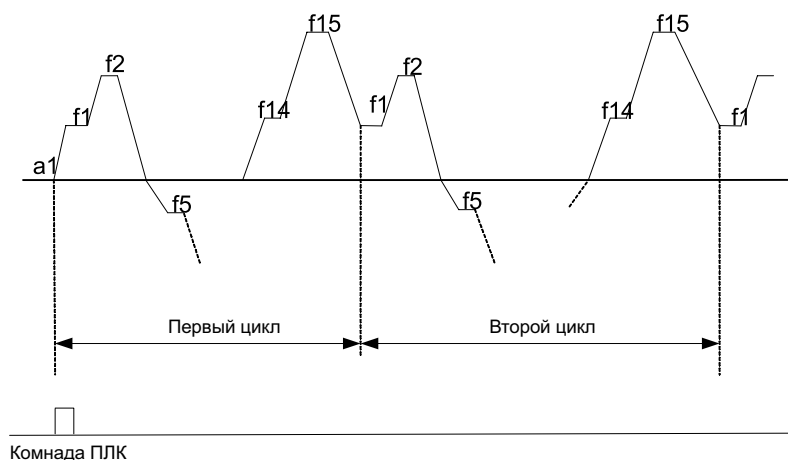
Рисунок 8.2.6. Режим непрерывного цикла при использовании простого ПЛК
