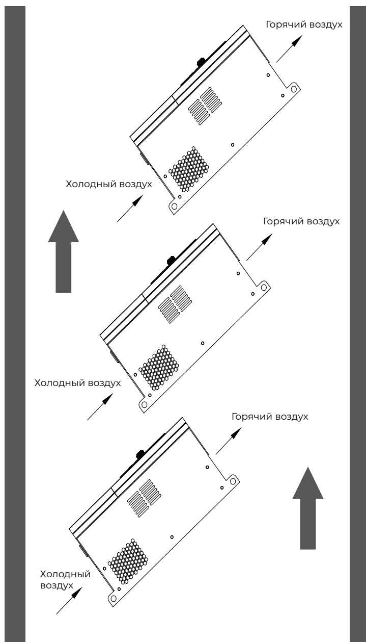
Рисунок 2.3. Наклонная установка нескольких преобразователей частоты
