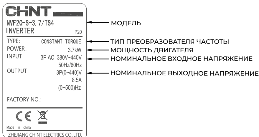
Рисунок 1.1. Заводская табличка устройства
