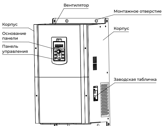
Рисунок 4.3. Внешние компоненты NVF2G-S-30/TS4-NVF2G-S-75/TS4
