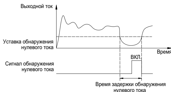
Рисунок 8.18.1. Принципиальная схема обнаружения нулевого тока
