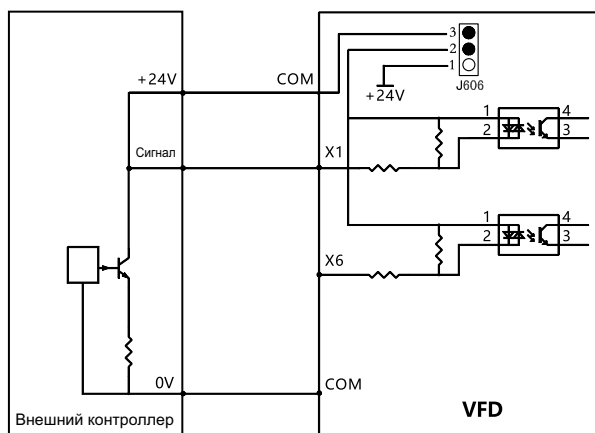
Рисунок 4.16. Схема подключения для логики NPN
