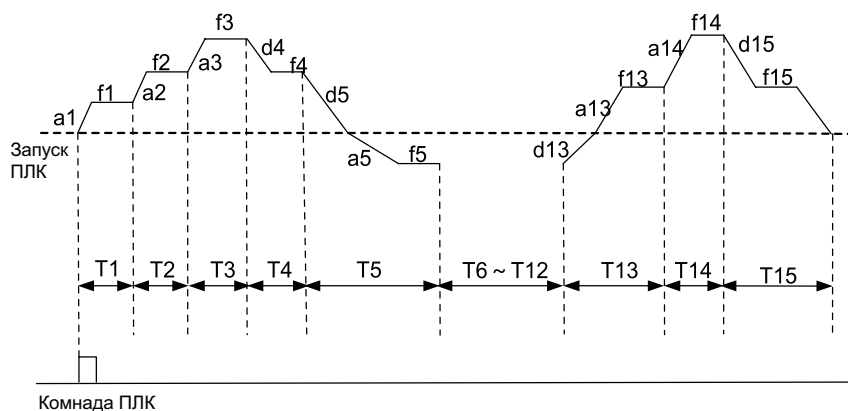
Рисунок 8.2.4. Режим останова после одного цикла при использовании простого ПЛК
