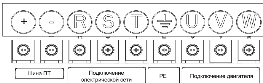
Рисунок 4.7. Силовые клеммы NVF2G-S-30/TS4-45/PS4
