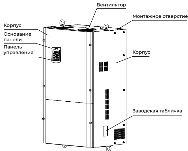
Рисунок 4.4. Внешние компоненты NVF2G-S-75/TS4–NVF2G-S-315/PS4
