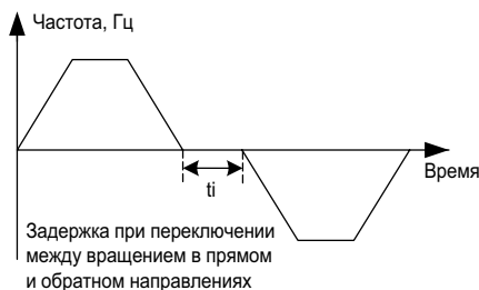
Рисунок 8.15.1. Принципиальная схема переключения между вращением в прямом и обратном направлениях
