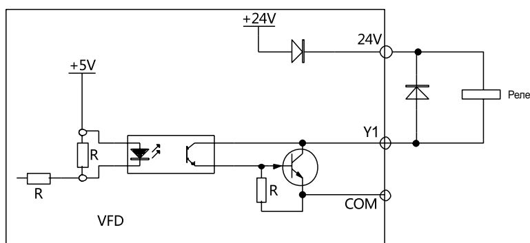
Рисунок 4.17. Схема подключения клеммы многофункционального выхода, режим 1
