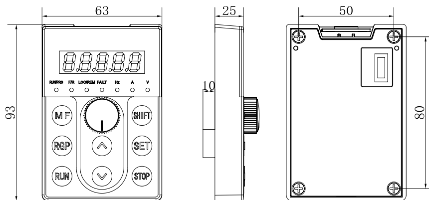
Рисунок 5.6. Панель управления
